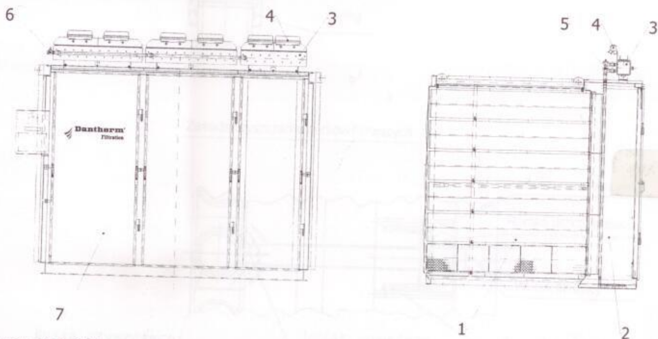
Rysunek 1. Główne zespoły odpylacza FD
